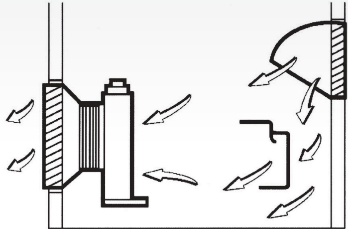
Şekil 7a. Örnek havalandırma sistemi - davlumnaz montajı çizimi
