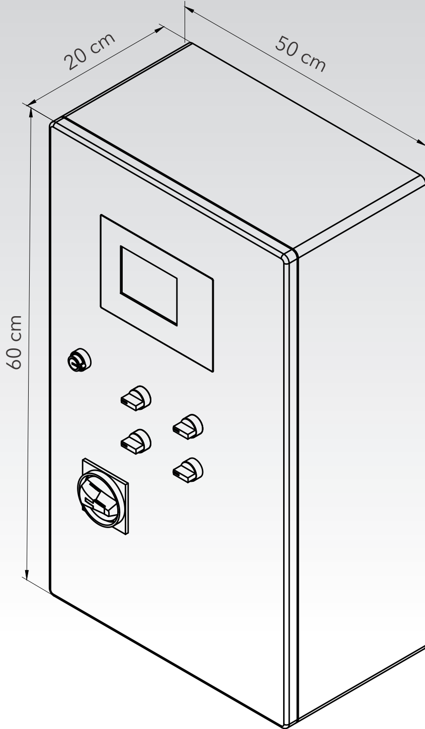
Şekil 2.1 Pano boyutları
