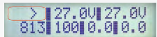
Şekil 9. Dize motor çalışıyor, basma kollektöründe basınç var (60 numaralı basınç kontrol klemensine basınç kontrol sensöründen gnd sinyali geliyor), rölanti süreci devam ediyor (dize düşük hızda çalışıyor)
