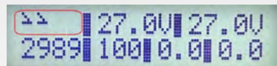
Şekil 8. Dize motor çalışıyor, basma kollektöründe basınç yok (60 numaralı basınç kontrol klemensine basınç kontrol sensöründen gnd sinyali gelmiyor), rölanti süreci bitti (dize yüksek hızda çalışıyor)
