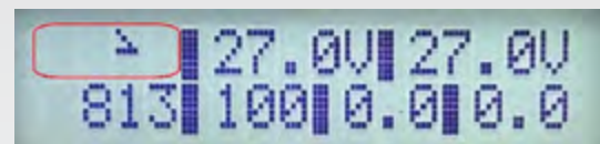
Şekil 7. Dize motor çalışıyor, basma kollektöründe basınç yok (60 numaralı basınç kontrol klemensine basınç kontrol sensöründen gnd sinyali gelmiyor), rölanti süreci devam ediyor (dize düşük hızda çalışıyor)
