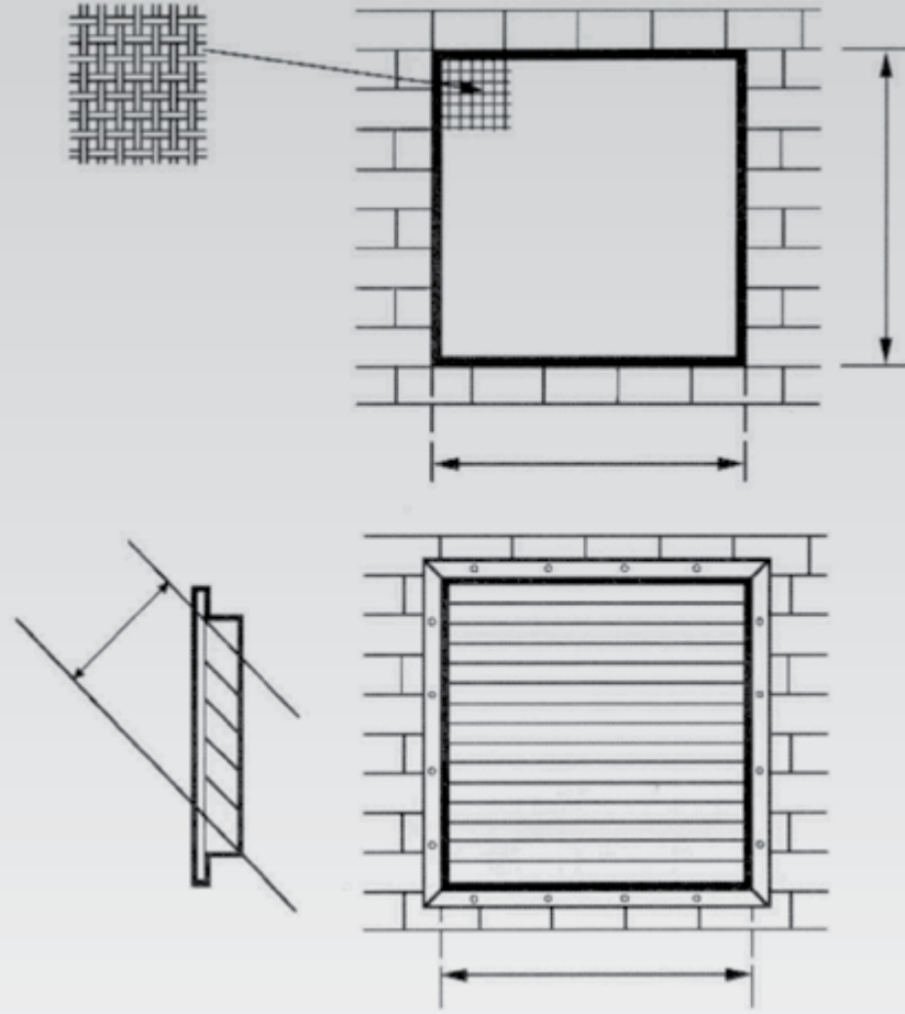
Şekil 46. Örnek radyatör menfez çizimi
