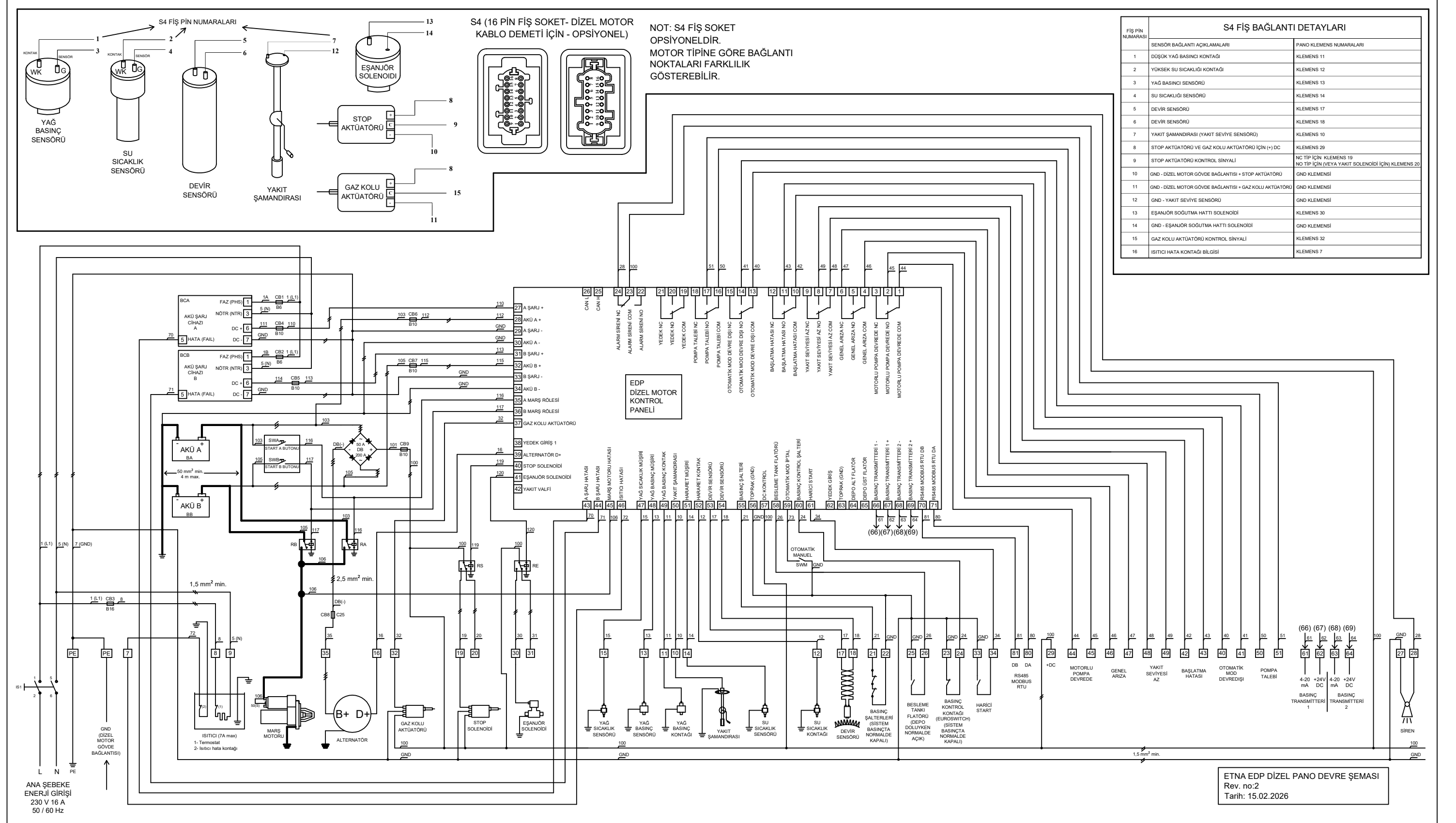
Şekil 48. EDP pano devre şeması
