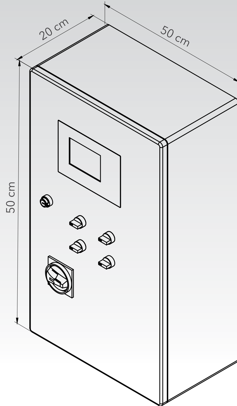
Şekil 2.1 Pano boyutları
