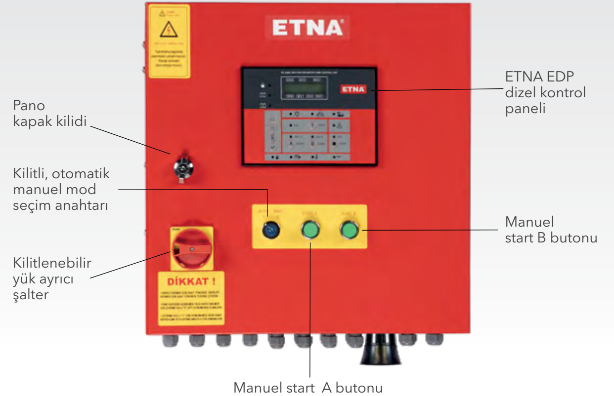
Şekil 1. ETNA EDP dizel pano dış görünümü
