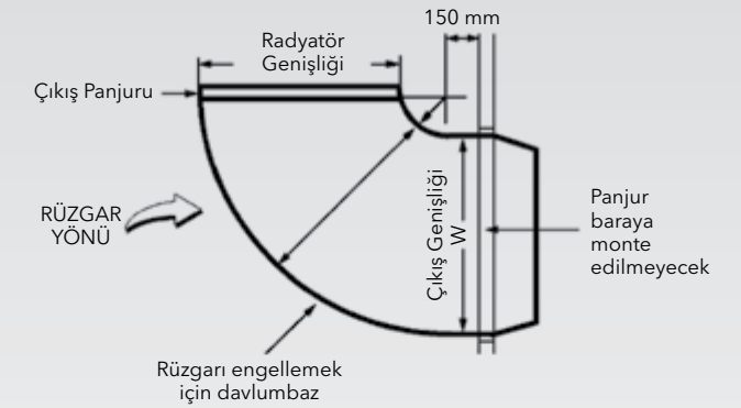
Şekil 46b. Örnek havalandırma sistemi - davlumbaz montajı çizimi
