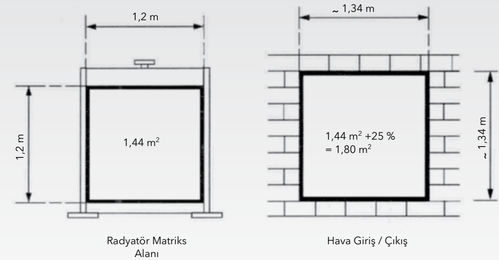
Şekil 45. Örnek Radyatör matriks alanı - havalandırma giriş hesabı
